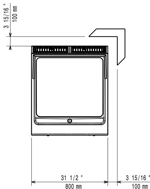
Felülnézet
